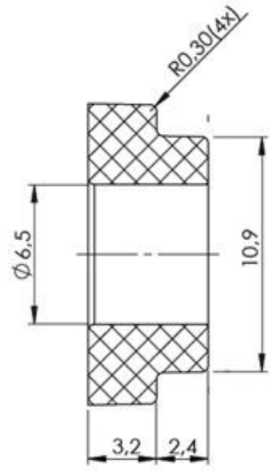
SEÇÃO A-A ESCALA 4 : 1
