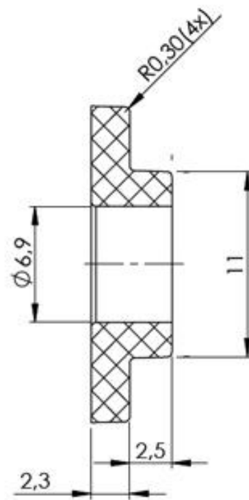
SEÇÃO A-A ESCALA 3 : 1
