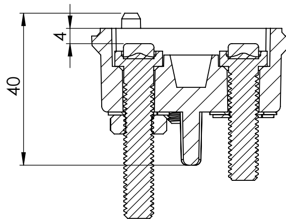
SEÇÃO A-A
