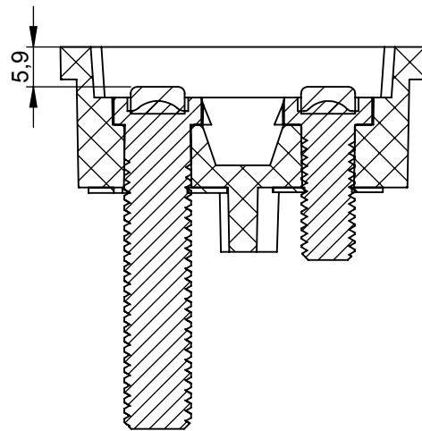
SEÇÃO A-A ESCALA 1 : 1
